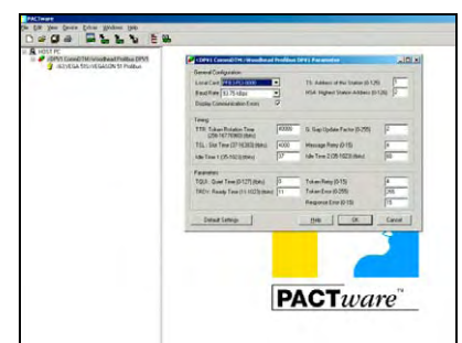
- Pactware Screenshot -
